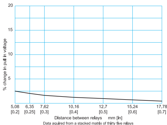
Fig. #8 Alternate Pairs Matrix.
